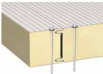
Płyta ścienna ze standardowym zamkiem
