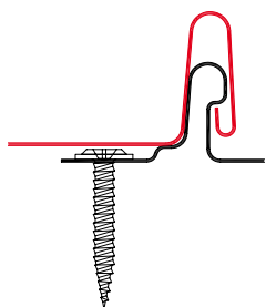
RYСУNEK 1. ZAMEK W PANELU DACHOWYM NA RĄBEK ELEGANT Z UKRYTYM MOCOWANIEM
