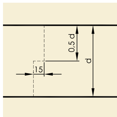
RYSUNEK 3. Połączenie frezowanych płyt BALEXTHERM SOFT
