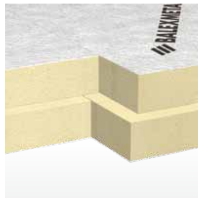
RYSUNEK 1. Płyta termoizolacyjna BALEXTHERM SOFT
