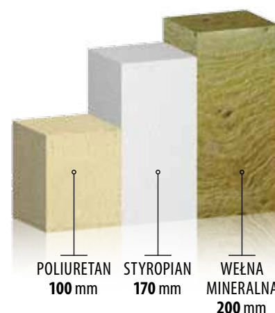
RYSUNEK 2. Grubość warstwy izolacyjnej wykonanej z różnych materiałów potrzebna do uzyskania współczynnika przenikania ciepła 0,22 W/m 2 K.
